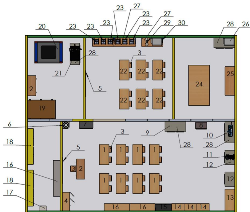
Рис. 1 План объекта
