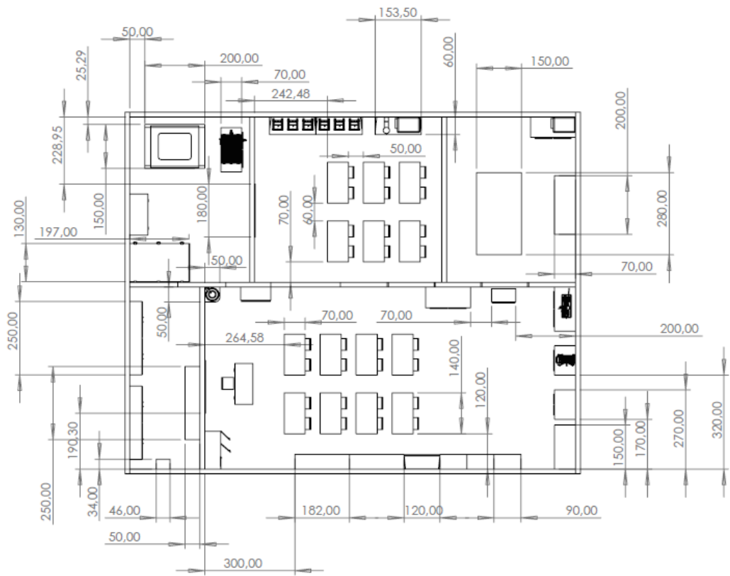
Рис. 3. Размерный план объекта 2
